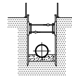
SECCION A-A
