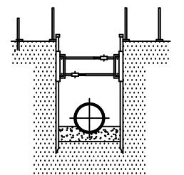
SECCION B-B
